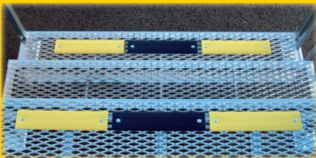
På nedre och övre steg (plattform) i trappa
